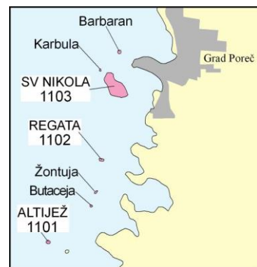
Kartogram akvatorija: 1:100.000
