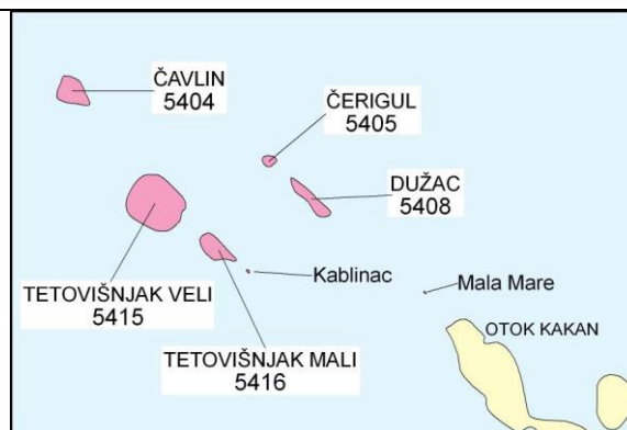
kartogram akvatorija 1:100.000
