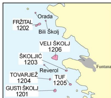
Kartogram akvatorija: 1:100.000
