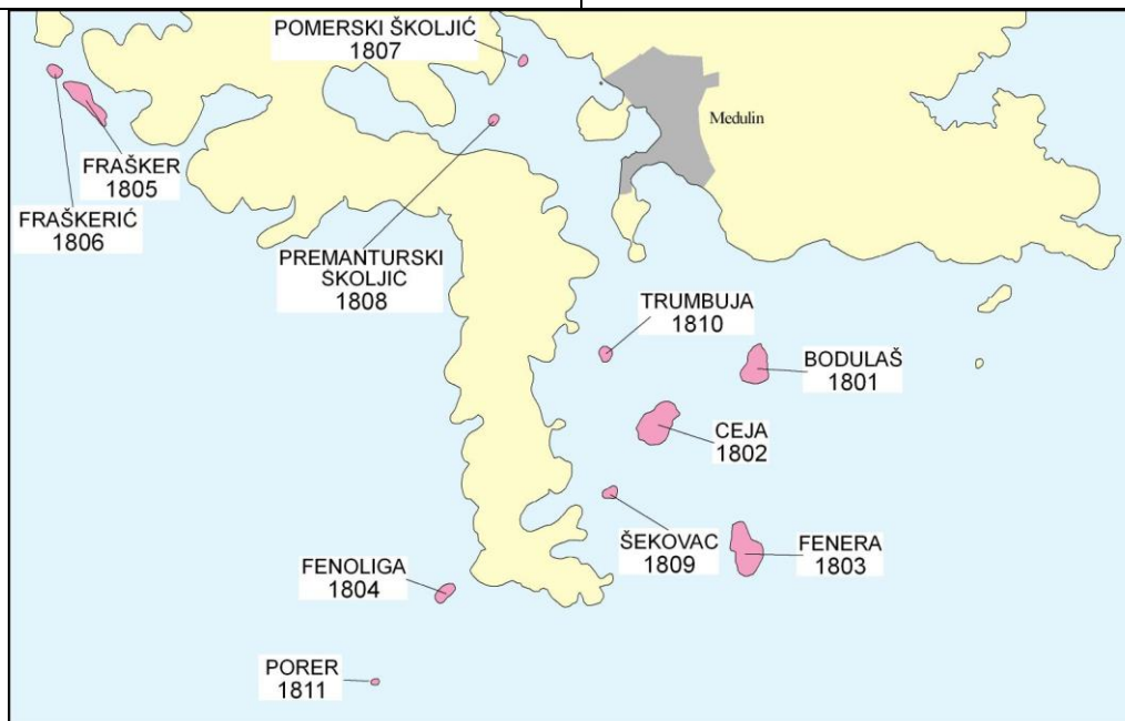
Kartogram akvatorija: 1:100.000
